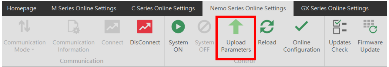
Fig 6. 3 Upload Parameters
